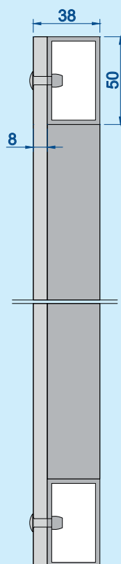
Przekrój pionowy w skali 1:3
