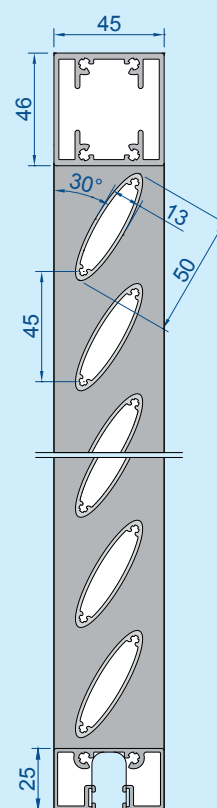
Przekrój pionowy w skali 1:3
