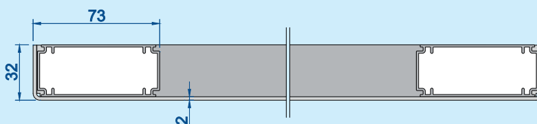
Horizontalschnitt: Maßstab 1:3
