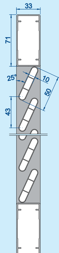
Vertikalschnitt: Maßstab 1:3
