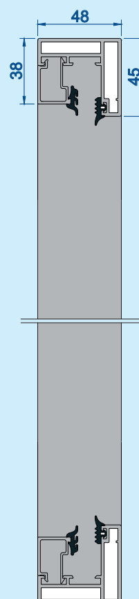
Przekrój pionowy w skali 1:3
