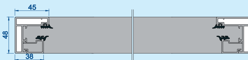
Przekrój poziomy w skali 1:3
